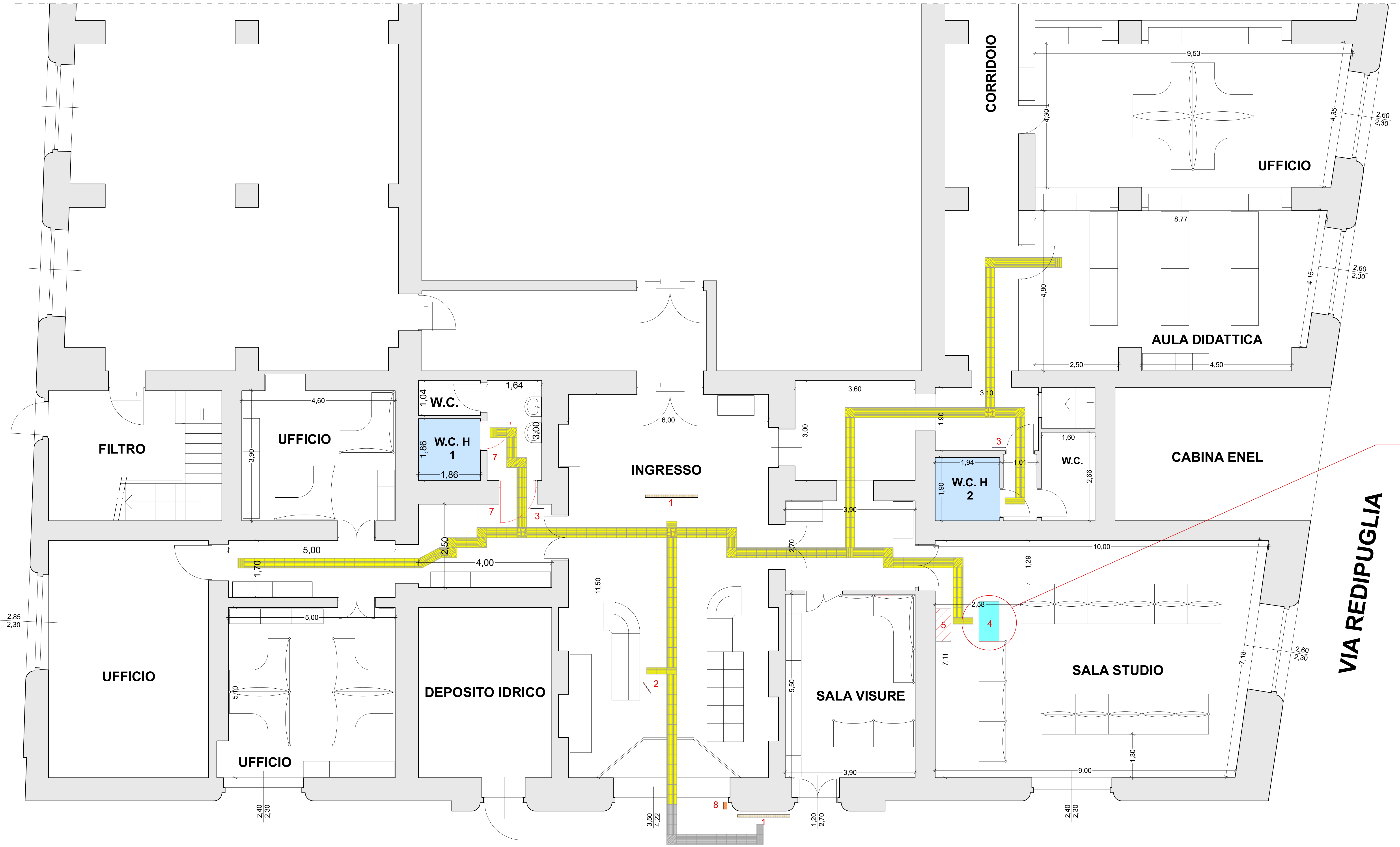
Pianta Piano Terra rapp. 1:50 Prime indicazioni strategiche
